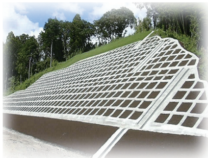
【国交省NETS登録・和歌山けんさんびん登録】 『SGフレーム工法軽量法枠やまChan』
