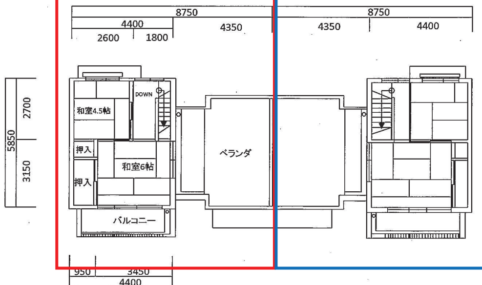
2 階 平 面 図
