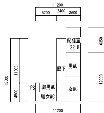
便所 1 階
