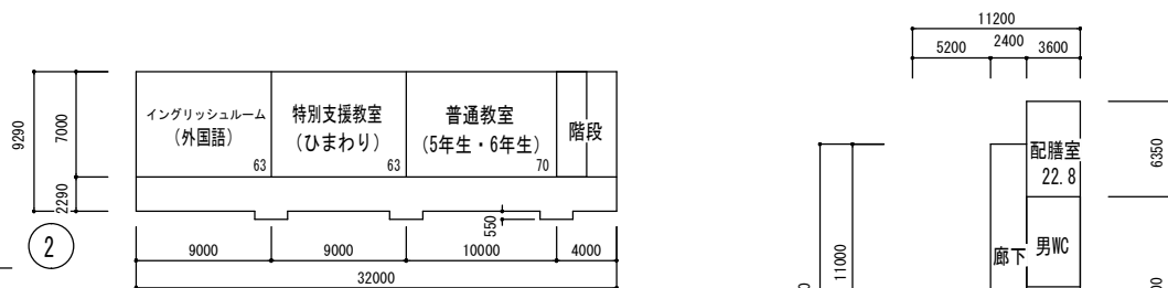
管理棟 2 階
