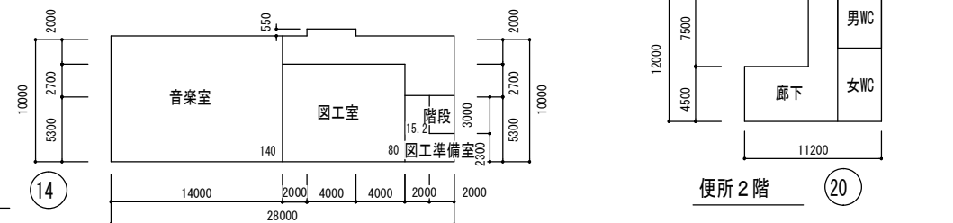
教室棟 3 階
