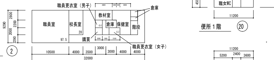
管理棟 1 階
