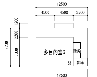
教室棟 1 階
