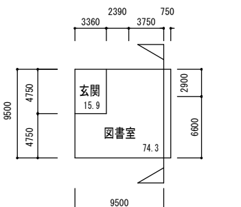
図書室 1 階
