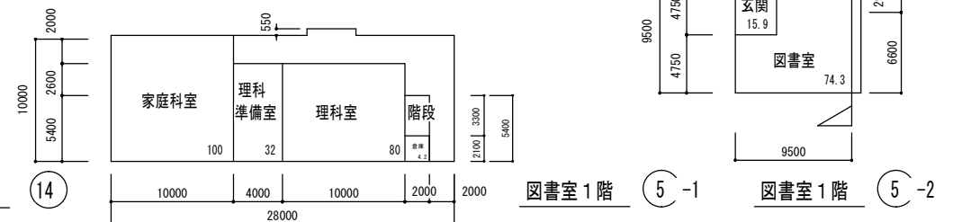
教室棟 1 階
