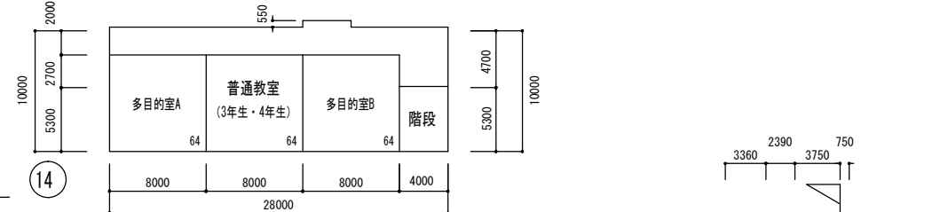
教室棟 2 階
