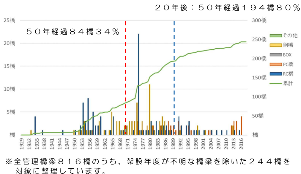
図 橋種ごとの架設年度
