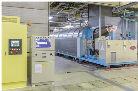
大型連続洗濯機
